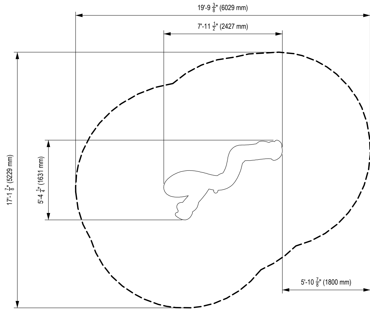
1 - CSA PLAN VIEW
